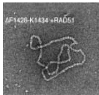
ADN au microscope électronique. Illustration extraite d'un article de Molecula Cell. , février 2001
